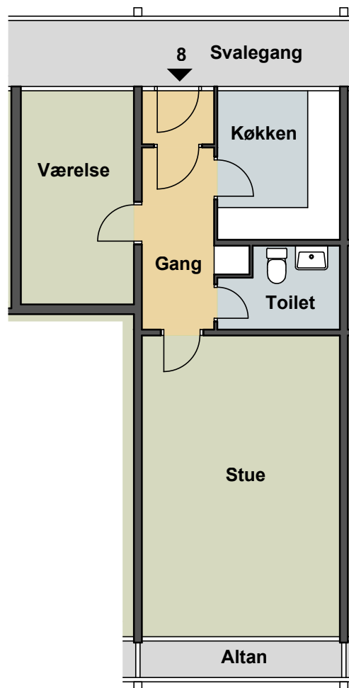
Plan 1:100
