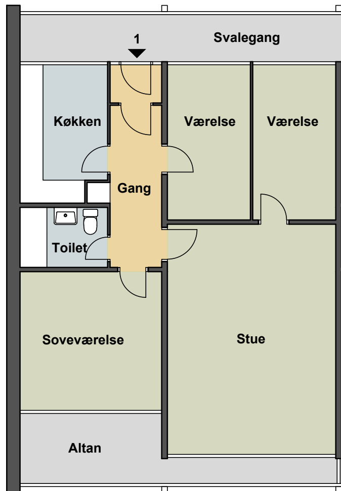
Plan 1:100
